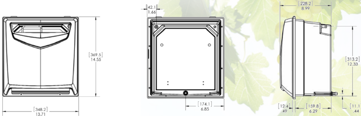
Vue de face, vue arrière et vue latérale Dimensions en pouces (mm)
