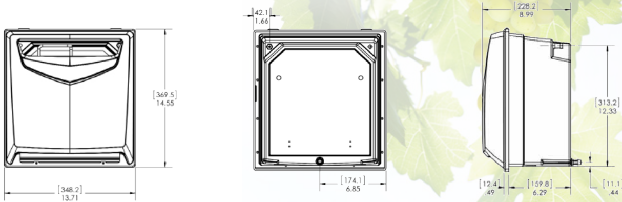
Vista frontal, posterior y lateral Dimensiones en pulgadas (mm)
