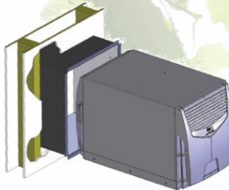
Vue latérale avec EasyMount™
